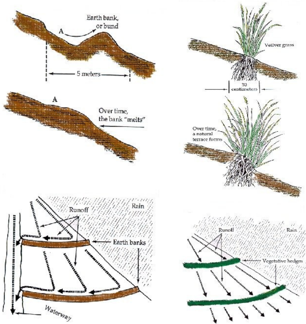
Gambar 1: Atas kiri: kontur tepian; kiri bawah: tepian mengalihkan air; kanan atas: pagar Vetiver membentuk tepian atau teras seiring waktu; kanan bawah: Pagar Vetiver memperlambat limpasan untuk meningkatkan perembesan, dan air tetap bertahan di ladang (Greenfield 1989)
