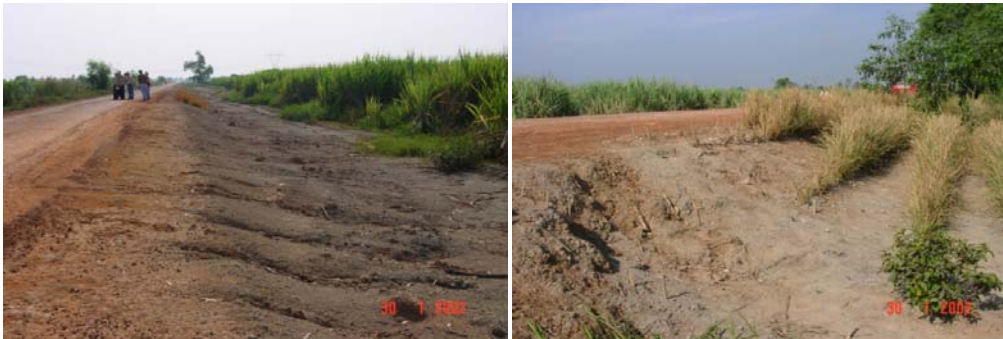
Foto 21: Sebelum dan sesudah penanaman Vetiver pada tanah ekstrim asam sulfat pada pematang di propinsi Tien Giang, Vietnam
