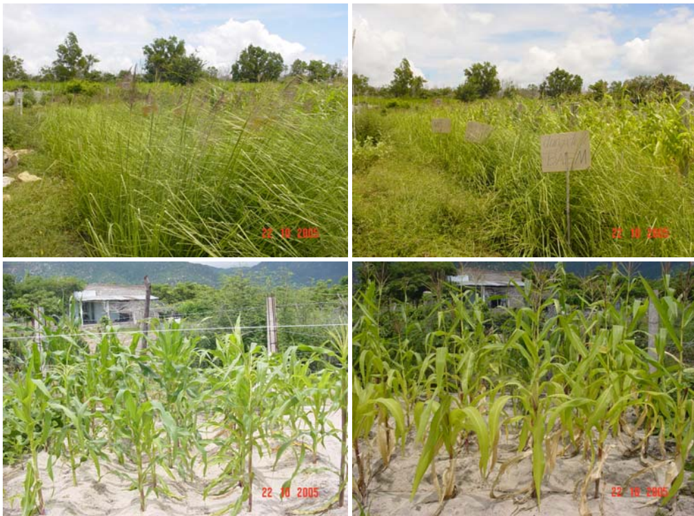
Foto 19: Akar Vetiver menghujam pembatas gipsum padat sampai air tanah dan tumbuh; tanpa irigasi jagung dan anggur mati
