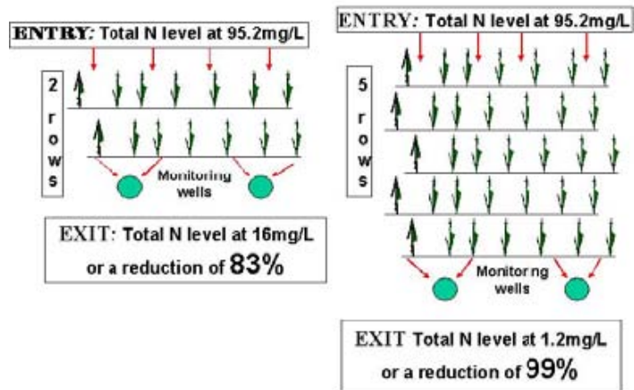
Gambar 4: Efektivitas pengurangan N pada limbah domestik
