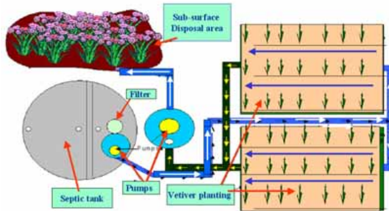
Gambar 5: Rancangan Sistem Pembuangan Domestik
