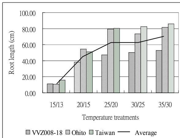
Gambar 1: Pengaruh suhu tanah terhadap pertumbuhan Vetiver
