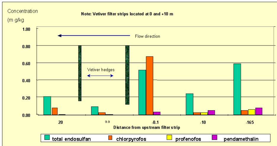
Gambar 3: Konsentrasi herbisida dalam tanah terkumpul di hulu dan hilir baris Vetiver penyaring
