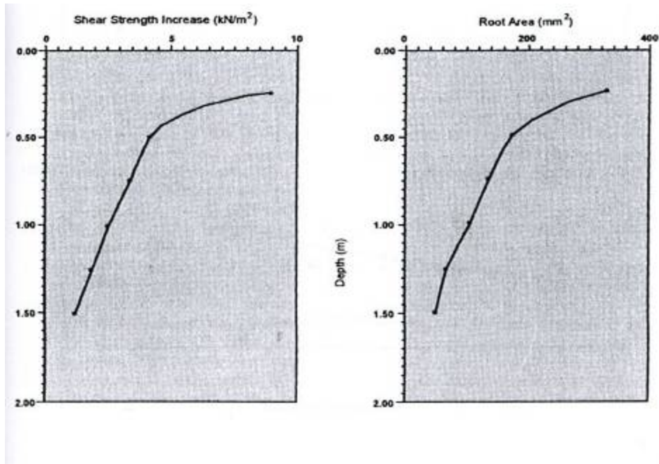
Gambar 3: Kekuatan geser akar Vetiver
